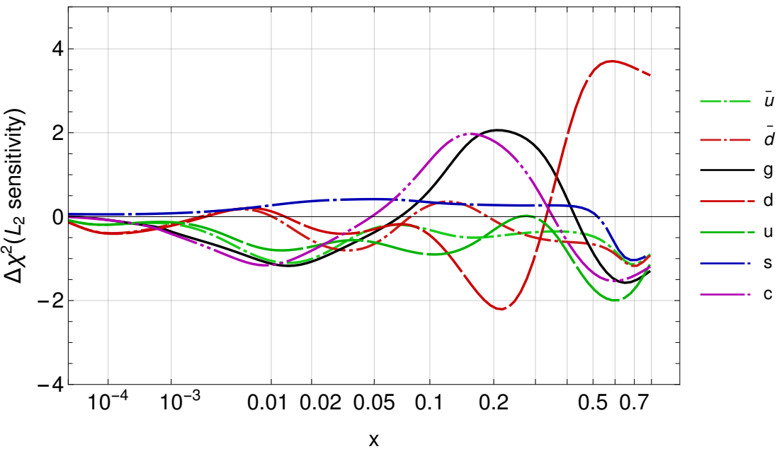
CT18Z NNLO, d02Easy5 (281), Q=2 GeV
